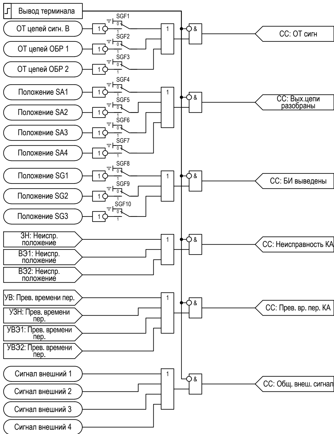
Рисунок 2.76 – Функциональная схема «СС»
