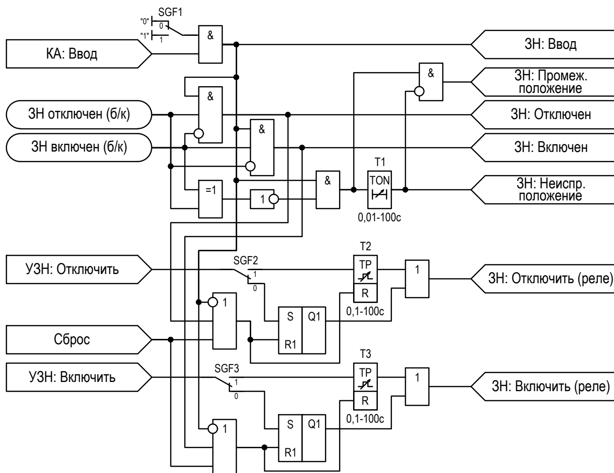
Рисунок 2.72 – Функциональная схема «ЗН»
