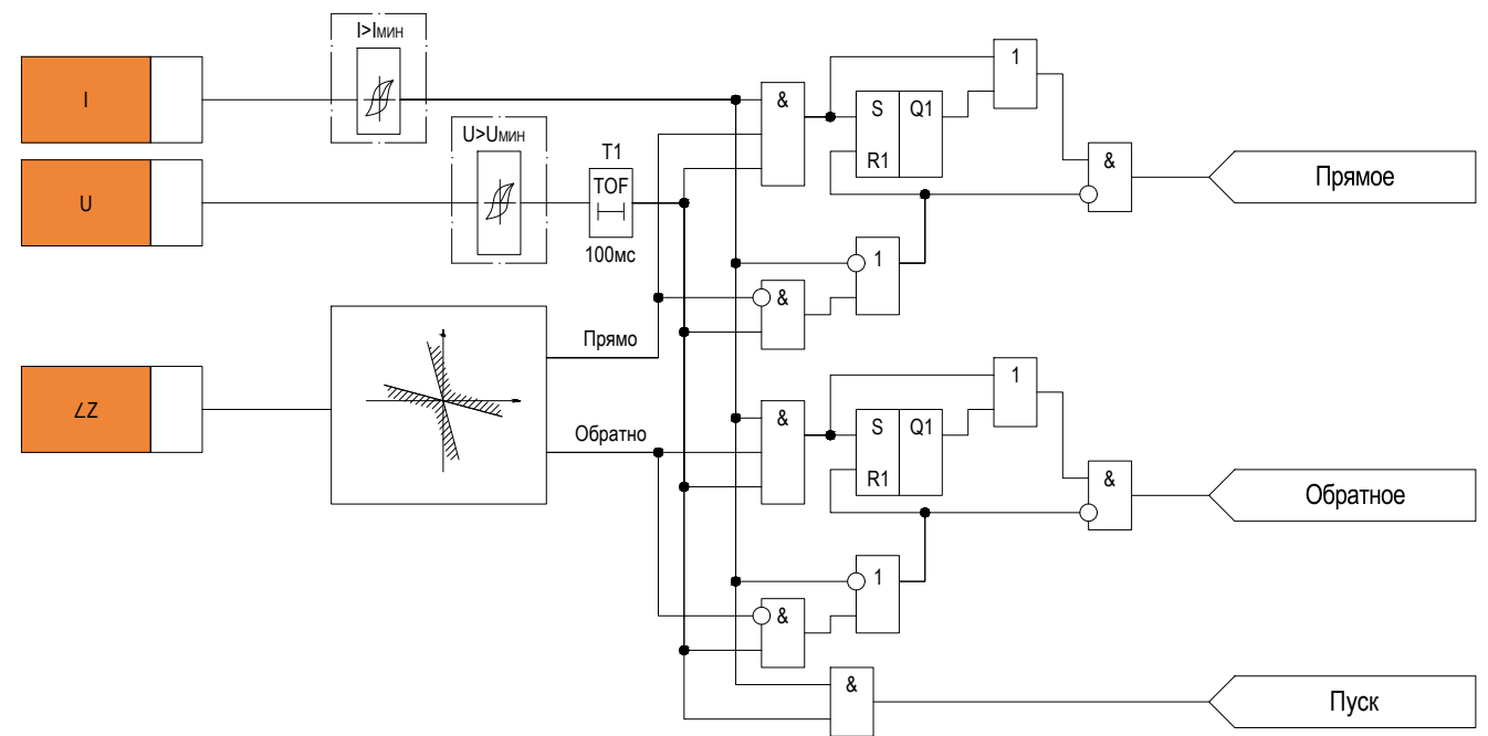
Рисунок 2.6 – Функциональная схема логики определения направления
