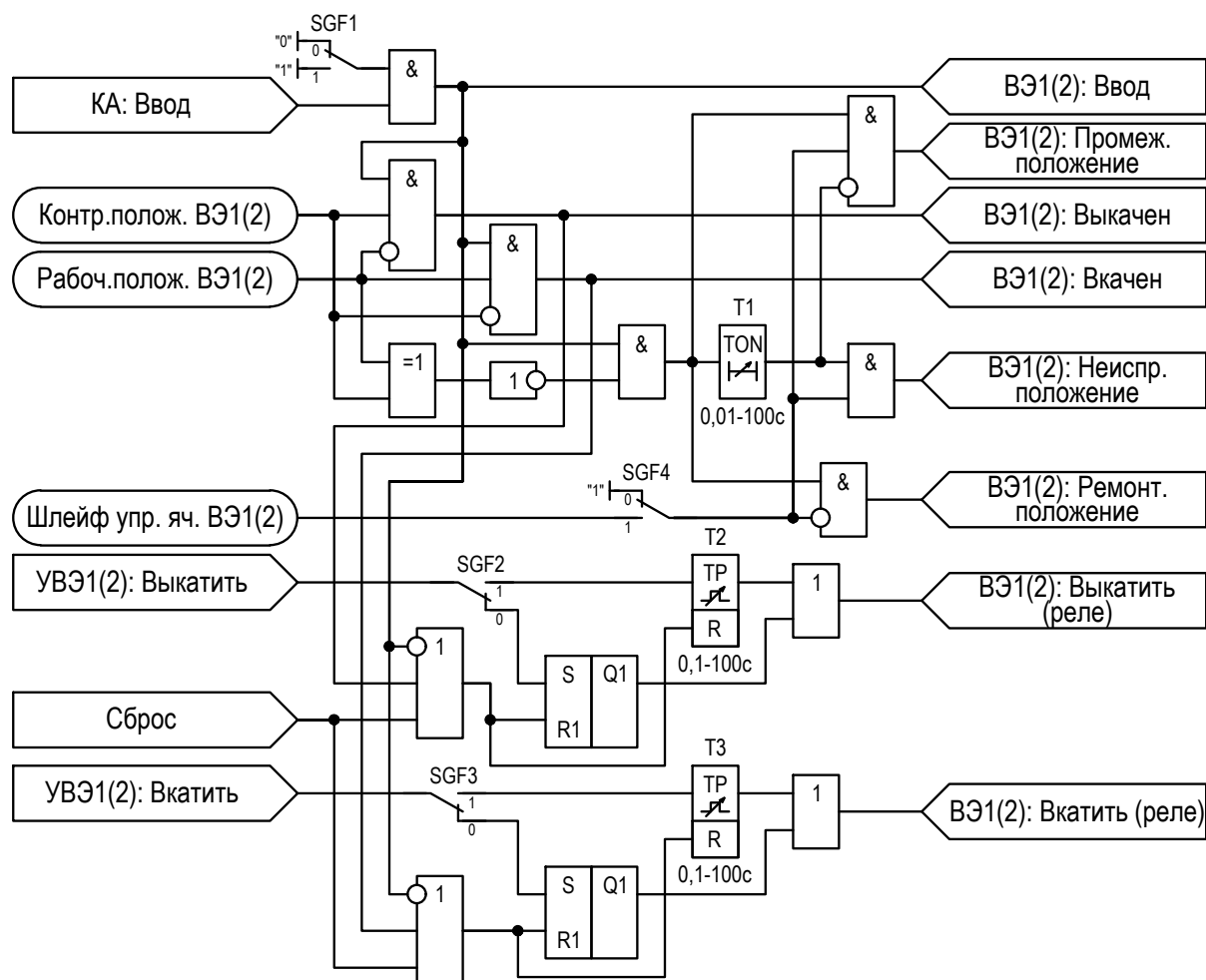
Рисунок 2.73 – Функциональная схема «ВЭ1(2)»
