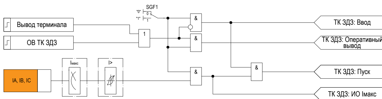
Рисунок 2.26 – Функциональная схема «ТК ЗДЗ»
